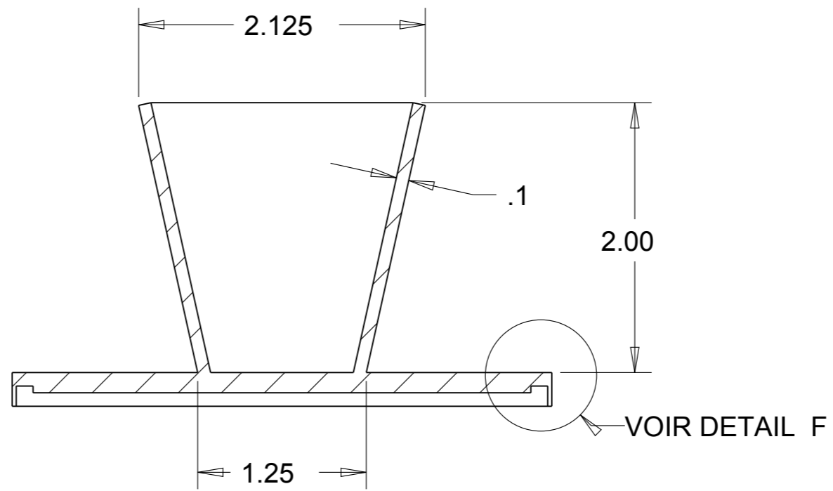
COUPE XSEC0001-XSEC0001
