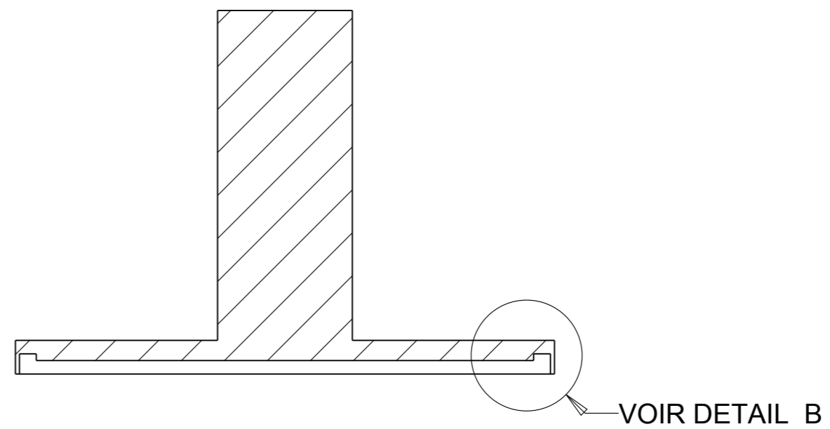
COUPE XSEC0002-XSEC0002
