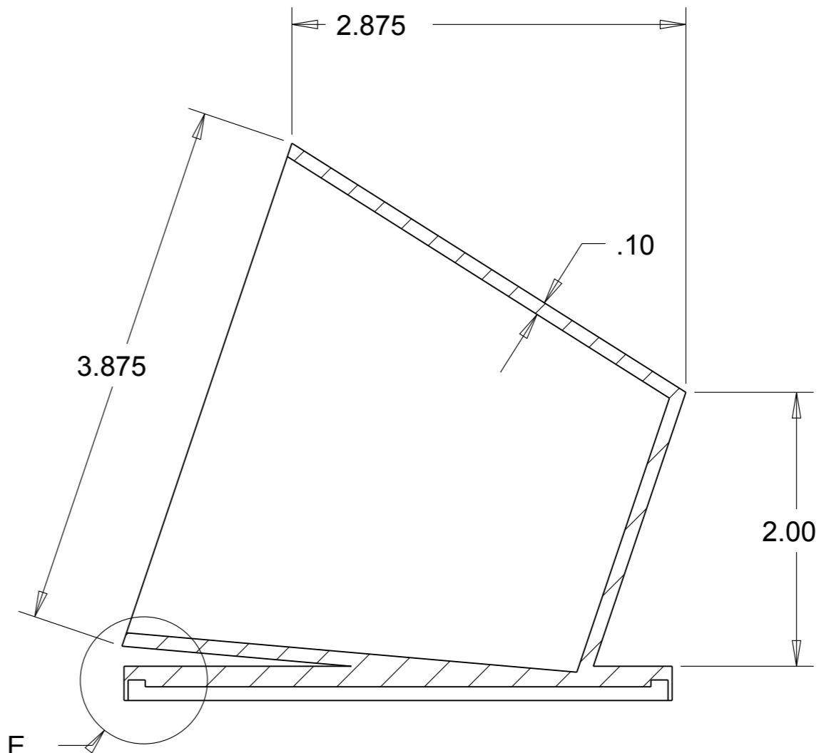
COUPE XSEC0002-XSEC0002
